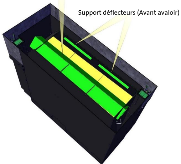
Support déflecteurs (Angle tuyère)
