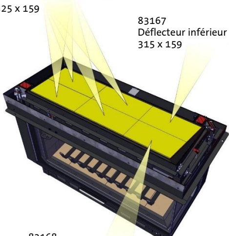
83168 Déflecteur inférieur latéral avant 309 x 159
