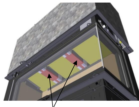
Boucliers thermique maintenu par 4 brides chacun
