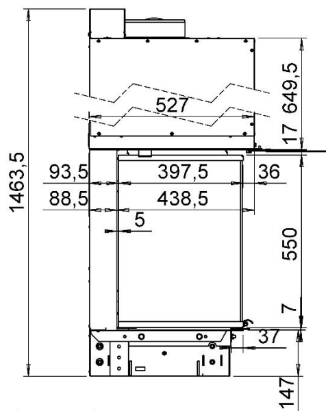
Coupe transversale
